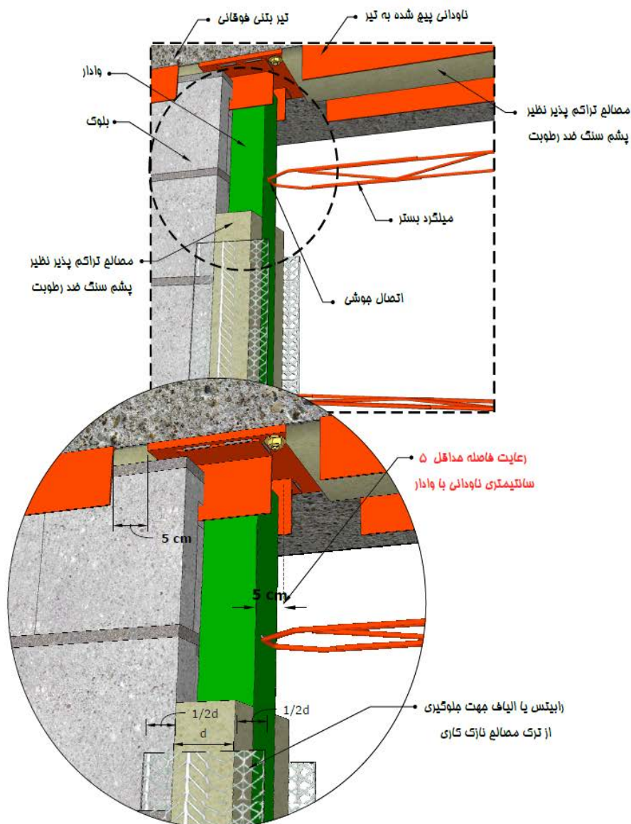
شکل پ ۴-۴- اجرای عایق پشم سنگ و مش الیاف یا رابطیس بر روی وادار
