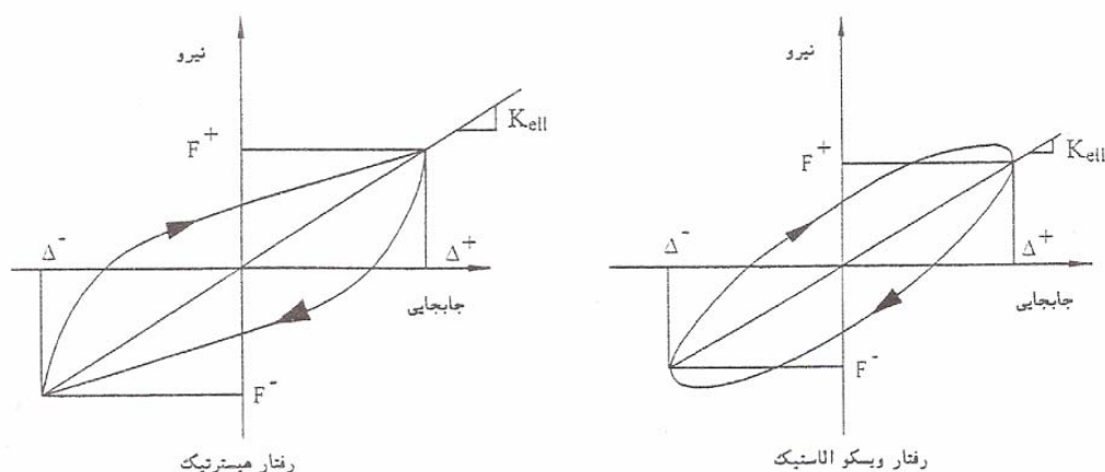
شکل (ت ۸-۱۰): سختی مؤثر جداسازهای لرزه‌ای
